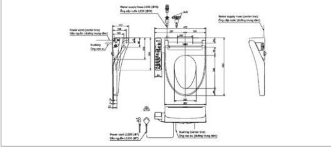
TCF2346OGAA TCF2341OGAA TCF2346OGAA Nắp rửa điện tử WASHLET
