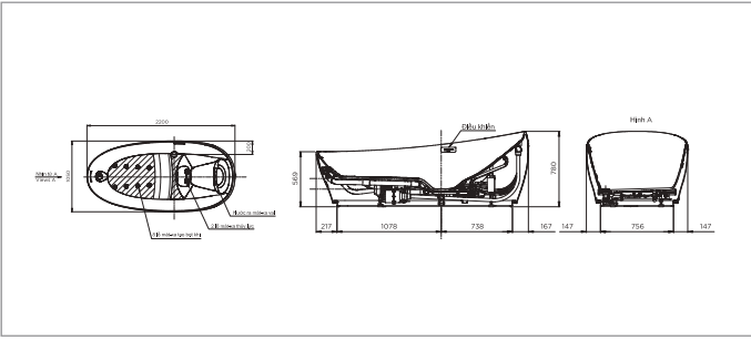
PJYD2200PWE PJYD2200PWE Bồn tắm nổi đặt sàn
