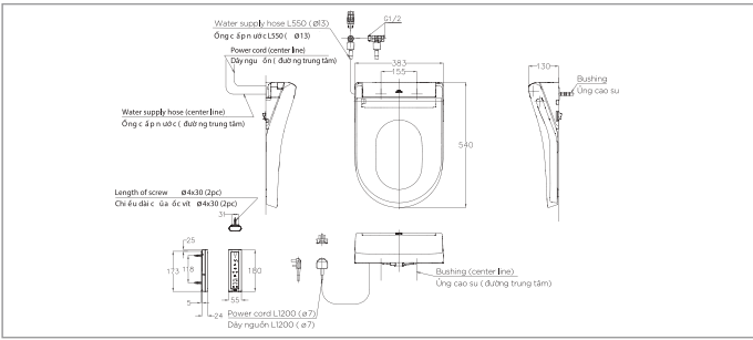
TCF3457OGAA TCF3432OGAA TCF3457OGAA Nắp rửa điện tử WASHLET
