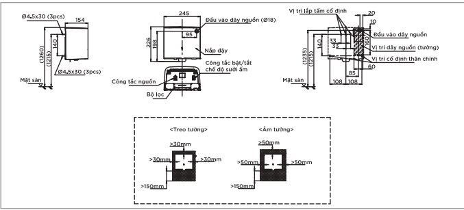
TYC322WF TYC122W TYC322WF TYC122W Máy sấy tay
