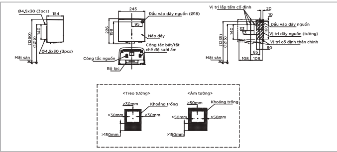
TYC322M TYC322M Máy sấy tay
