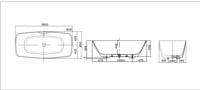
PJY1804HPWE PJY1804HPWE Bồn tắm GAGALATO đặt sàn
