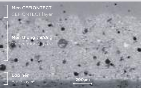
Men CEFIONTECT dưới kính hiển vi CEFIONTECT toilet micrograph *1Qm=0,001mm
