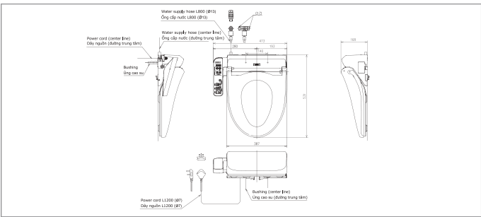
TCF2371OGAA TCF2371OGAA Nắp rửa điện tử WASHLET
