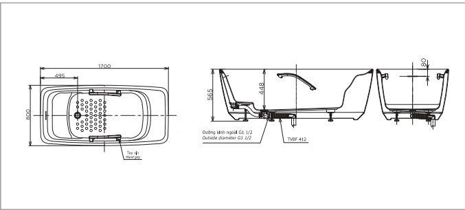
PJY1724HPWE PJY1724PWE PJY1724HPWE Bồn tắm GAGALATO đặt sàn Bao gồm tay vịn PJY1724PWE Không bao gồm tay vịn
