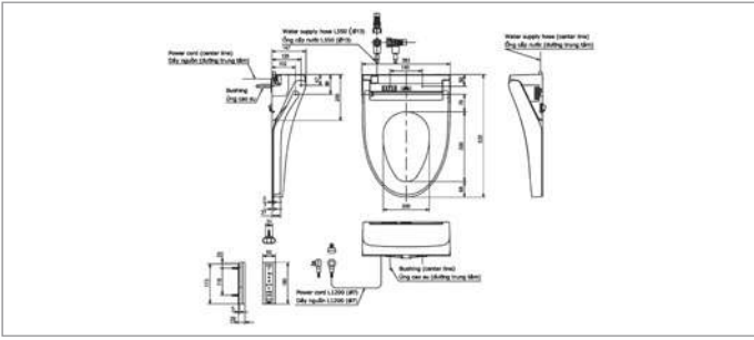
TCF2446OGAA TCF2441OGAA TCF2446OGAA Nắp rửa điện tử WASHLET
