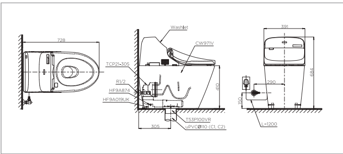
C971P TCF9433A C971P TCF9433A Thân cầu Nắp rửa điện tử
