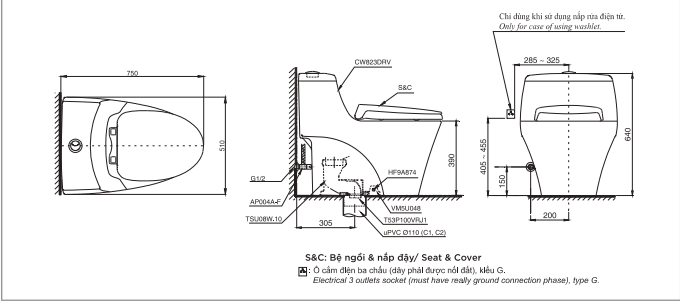
MS823DRT2 CW823DRV Thân cầu
