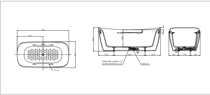
PJY1734HPWE PJY1734PWE PJY1734HPWE Bồn tắm GAGALATO đặt sàn Bao gồm tay vịn PJY1734PWE Không bao gồm tay vịn
