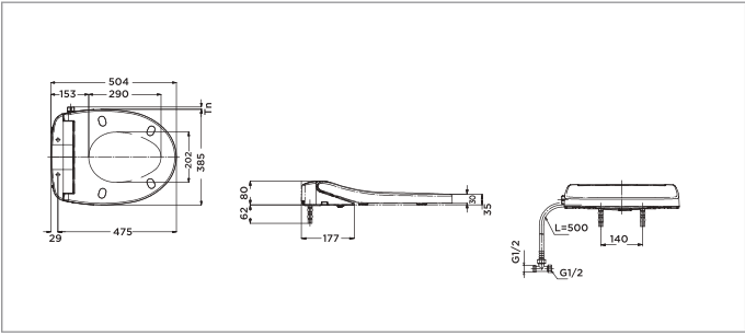
TCW07S TCW07S Nắp rửa cơ Ecowasher
