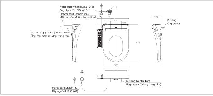
TCF3337OGAA TCF3332OGAA TCF3337OGAA Nắp rửa điện tử WASHLET
