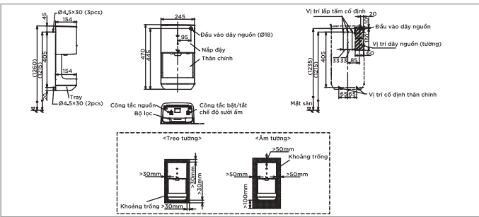
TYC322W TYC322W Máy sấy tay
